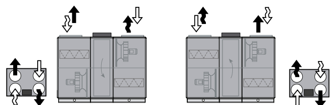
Ventilatorstand 1 ingesteld als inlaatlucht (inspectiezijde links)
