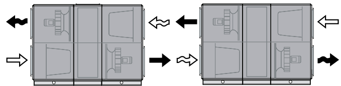
Ventilatorstand 1 ingesteld als uitlaatlucht (inspectiezijde rechts)
