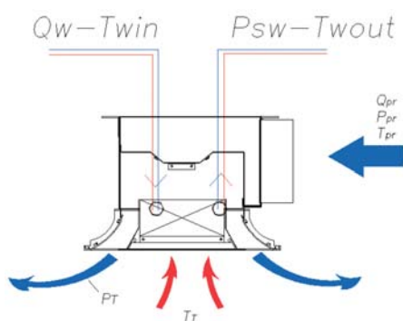
Systeem 2 leidingen
