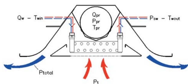
Systeem 2 leidingen
