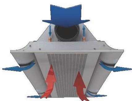
Detail werkingsprincipe
